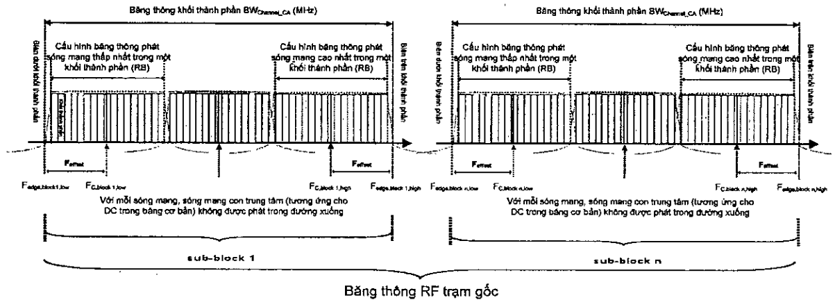
Hình 3 – Băng thông khối thành phần cho phổ không liên kề nội băng tần
