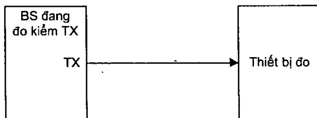
Hình C.1 – Thiết lập hệ thống đo công suất ra của trạm gốc, công suất ra động, chất lượng tín hiệu phát, lỗi tần số, EVM, công suất DL RS, phát xạ không mong muốn
