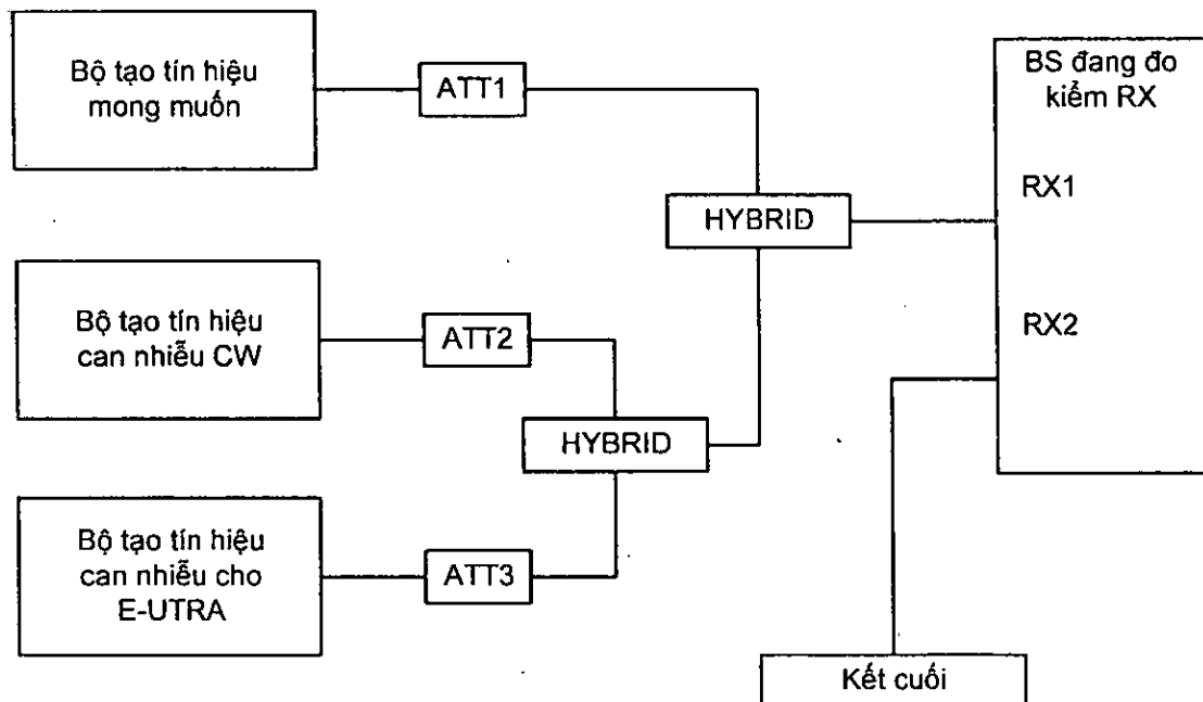
Hình C.13 – Thiết lập hệ thống đo các đặc tính xuyên điều chế
