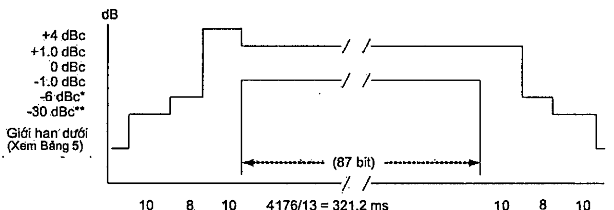
Hình C.2 - Mẫu công suất/thời gian đối với cụm truy nhập
