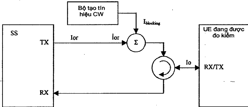
Hình B.6.4 - Sơ đồ đo kiểm RX với CW bổ sung
