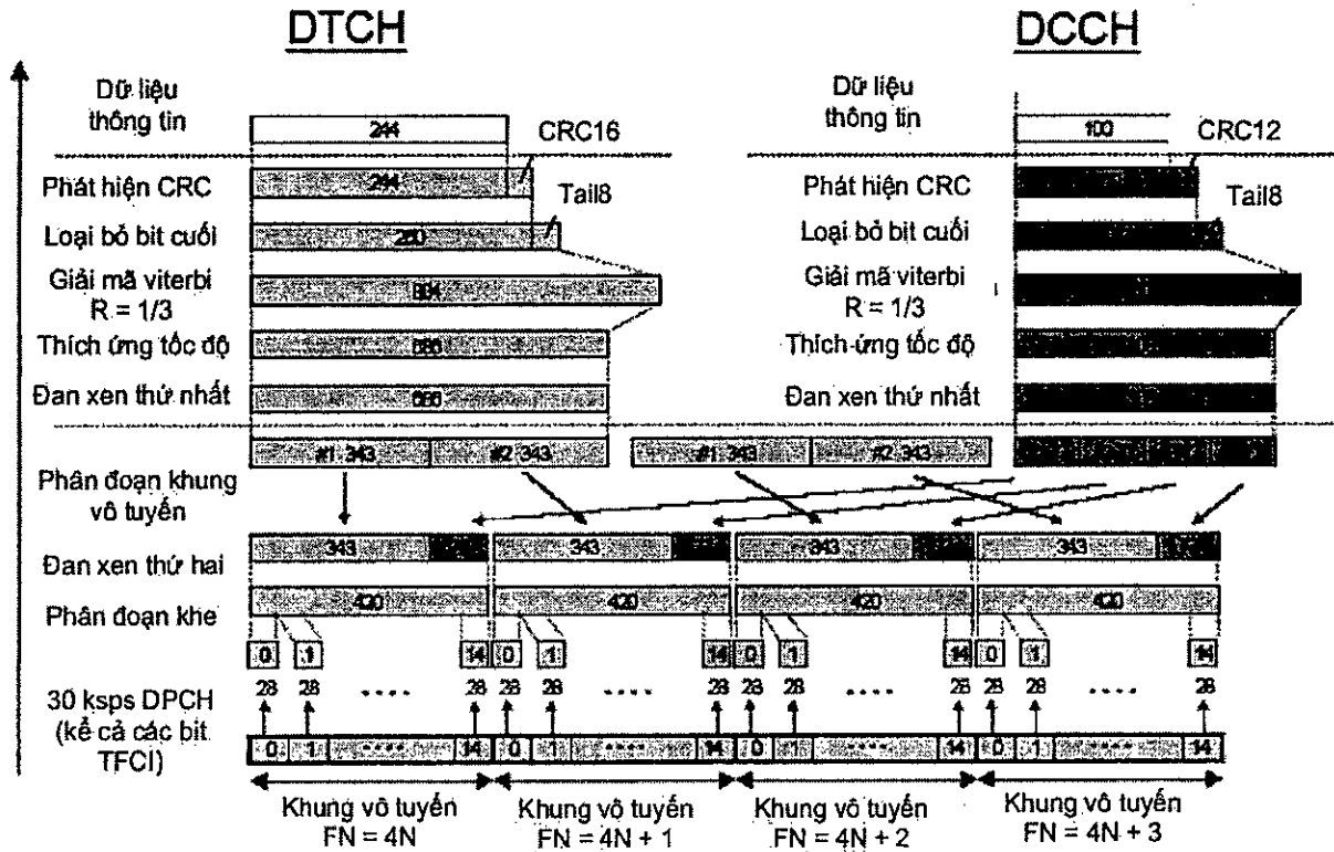
Hình B.7.1.1 - Mã hoá kênh đo tham chiếu DL (12,2 ki/s)
